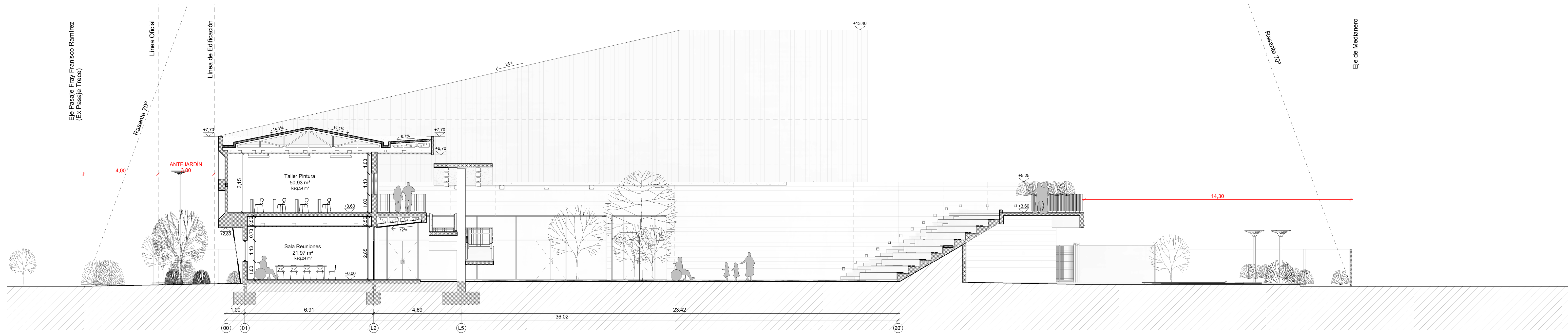
Sección A-A' Escala 1 : 100
