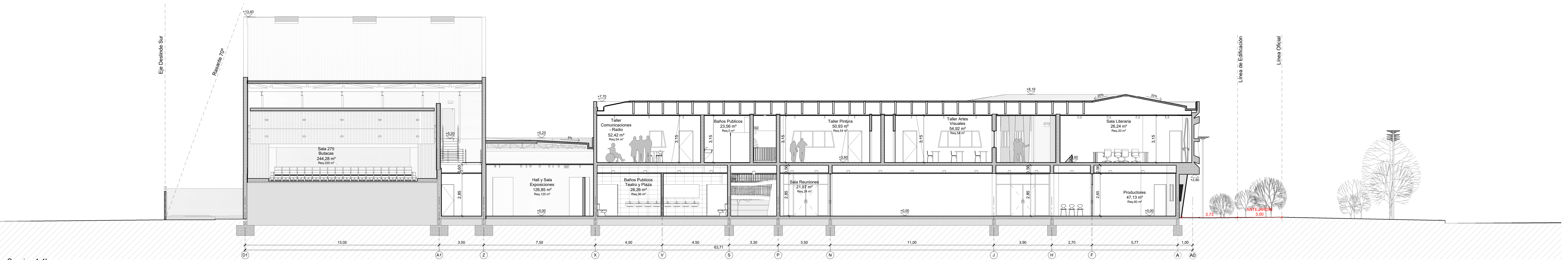
Sección 1-1' Escala 1 : 100
