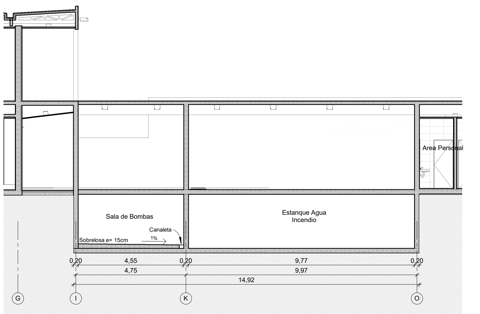
Corte A-A' Estanque Escala 1 : 100
